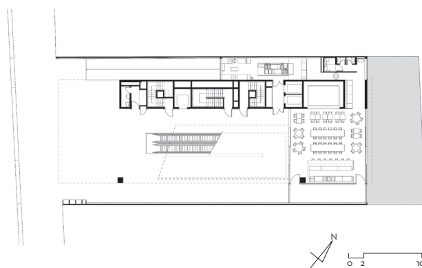
ERDGESCHOSS | REZ-DE-CHAUSÉE
