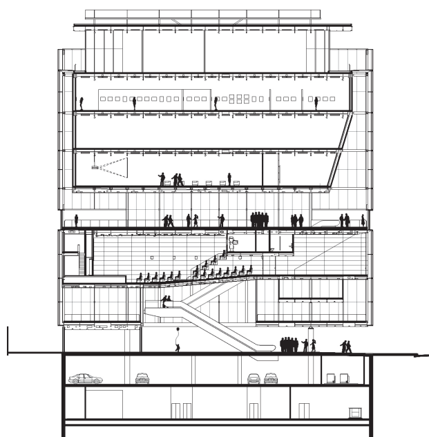
LÄNGSSCHNITT | COUPE LONGITUDINALE
