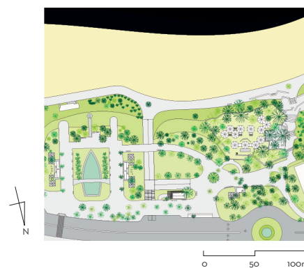
LAGEPLAN | PLAN DE SITUATION
